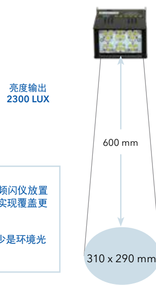
距离600MM处， 聚光型的覆盖范围
