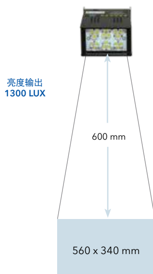
距离600MM处， 泛光型的覆盖范围
